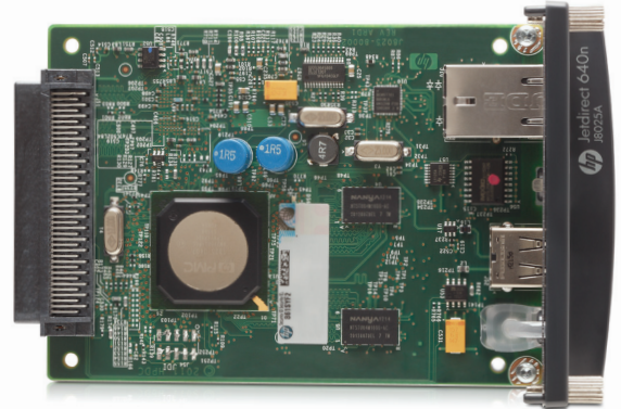
HP Jetdirect 640n Print Server
